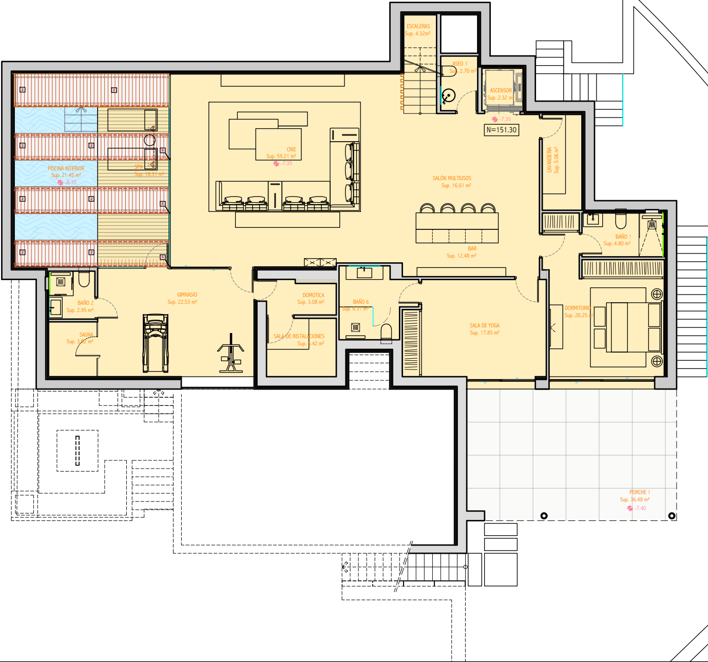
PLANTA SOTANO SUPERFICIE CONSTRUIDA: 278.87m2
