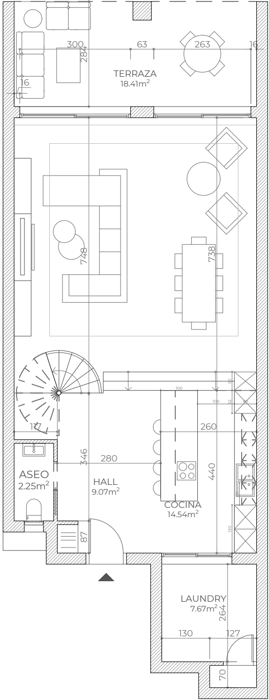
PLANTA BAJA
